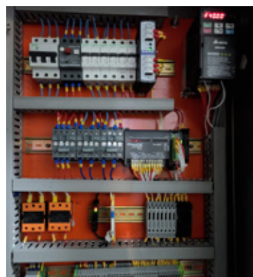
Cableado de tablero eléctrico fuerza y control (Empresa Ittem SAC)
